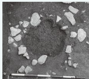
石囲いの炉跡(縄文時代後期) 炉跡の実測図
